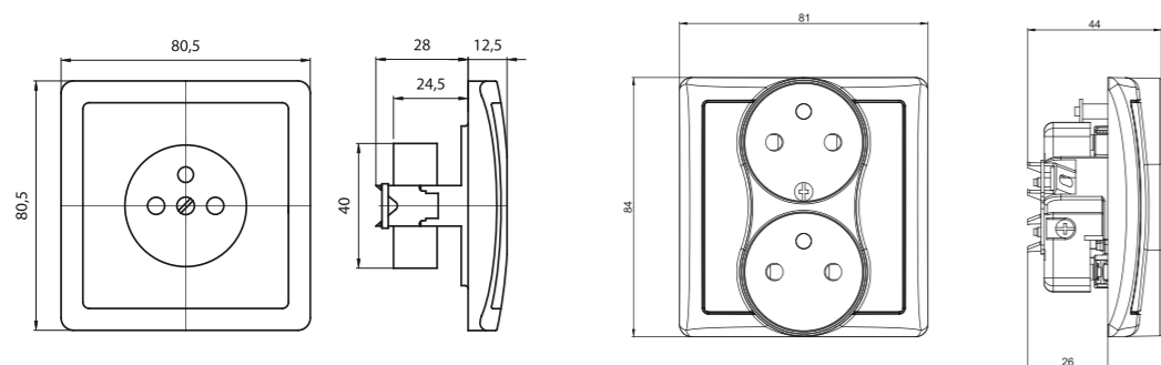
Zásuvka jednonásobná a zásuvka dvojnásobná
